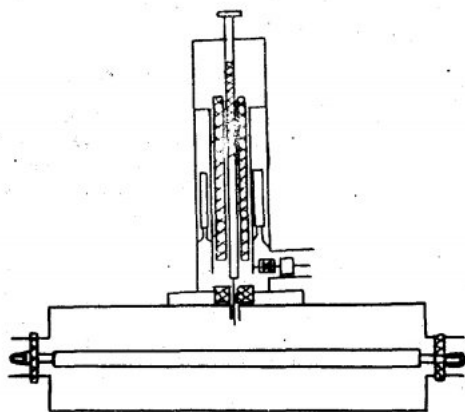
Рисунок 2 – схема измерительной линии
