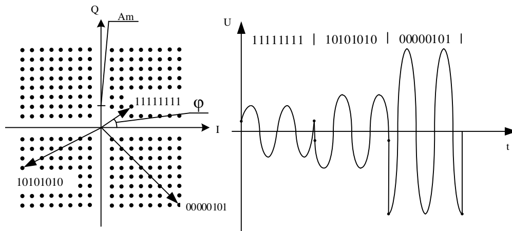
Рисунок 2 – Пример типовой временной диаграммы сигнала QAM-256
