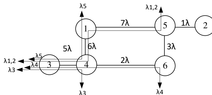
Рисунок 4 – Пример разметка оптических каналов связи узла 3 с другими узлами связи WDM Последующая разметка каналов связи с узлами WDM выполняются аналогично. Так, для участка
