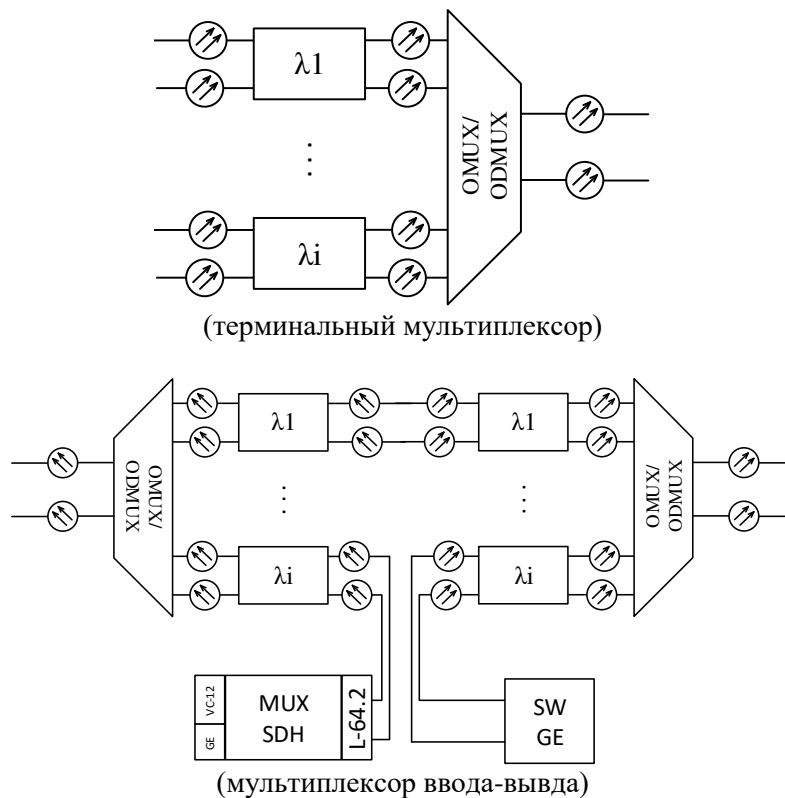
Рисунок 2 – Схема сетевого узла WDM
