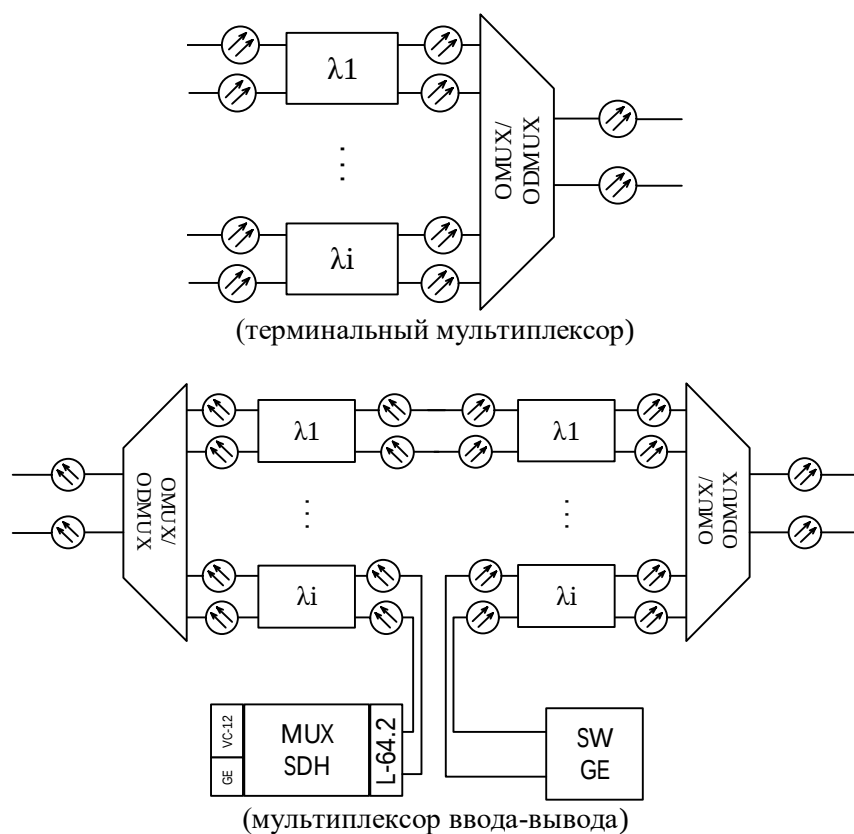
Рисунок 2 – Схема сетевого узла WDM
