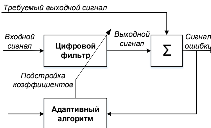
Рис. 1– Обобщенная структурная схема одноканального адаптивного фильтра
