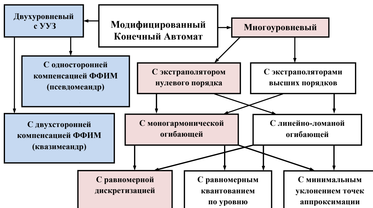
Рис. 2. Классификация МКА по способу реализации выходной частоты
