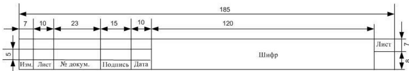
Рисунок Г.2 - Штамп листов пояснительной записки текстового документа
