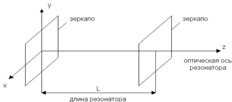
Рисунок 1 - Резонатор Фабри-Перо
