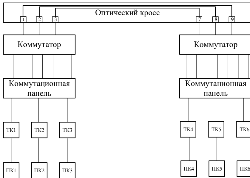
Рисунок 4.1 – Схема монтажа структурированной кабельной системы
